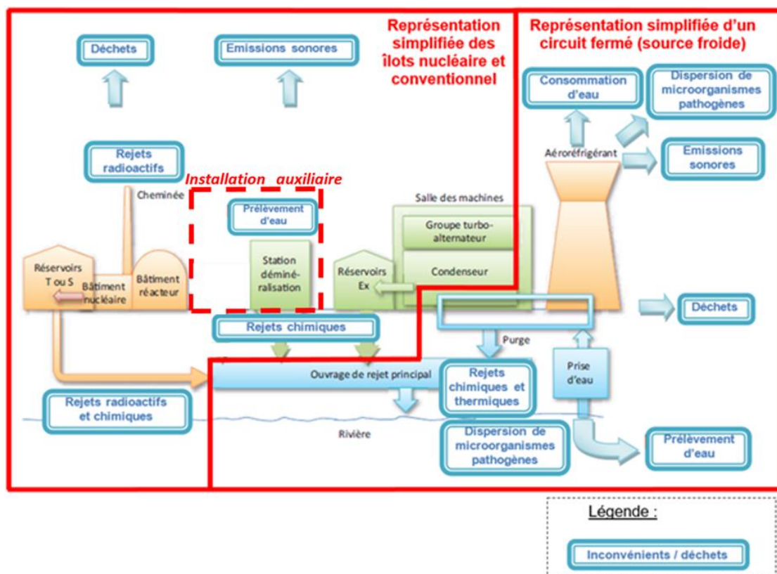
Figure 35 : Présentation schématique des îlots nucléaire et conventionnel et de la source froide ainsi que des inconvénients associés (CNPE refroidi en circuit dit « fermé »)
